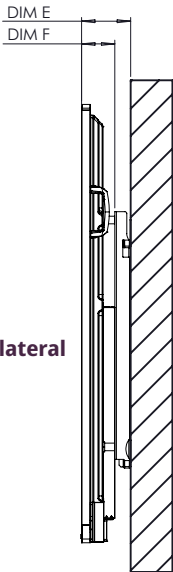
Vista lateral
