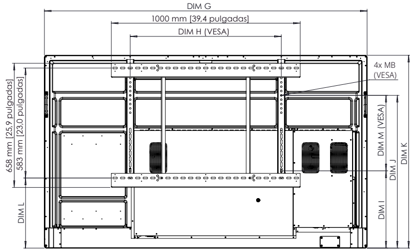
Vista posterior
