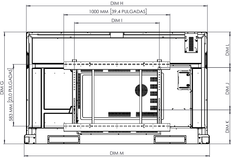
Parte posterior
